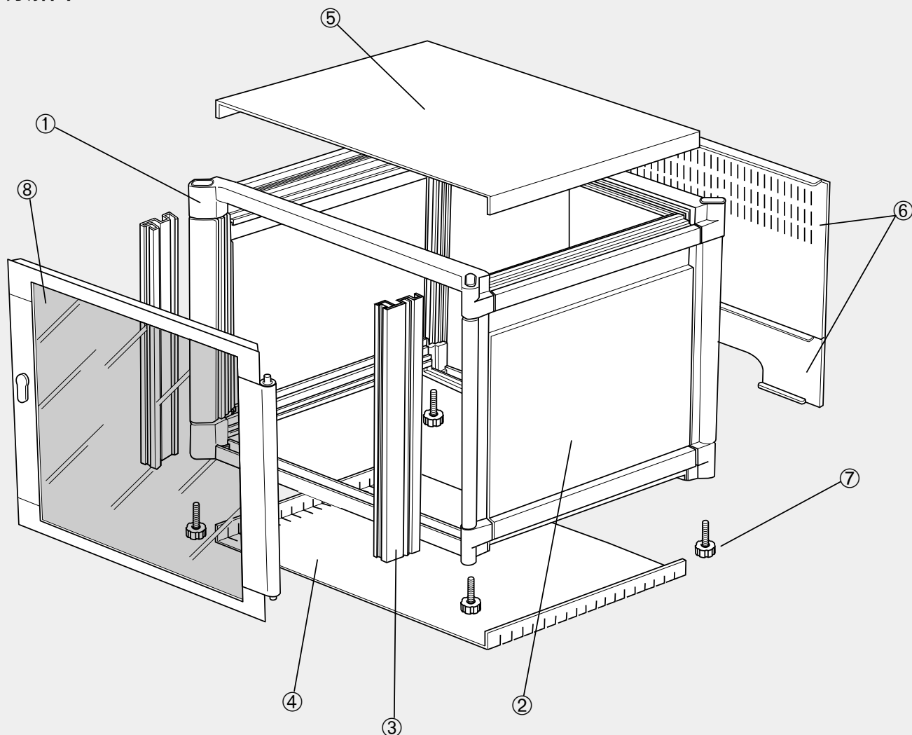
分解図
