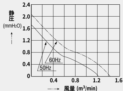
データ（風量－静圧特性）
