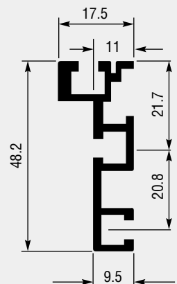
フロント・リヤパネルマウントフレーム
