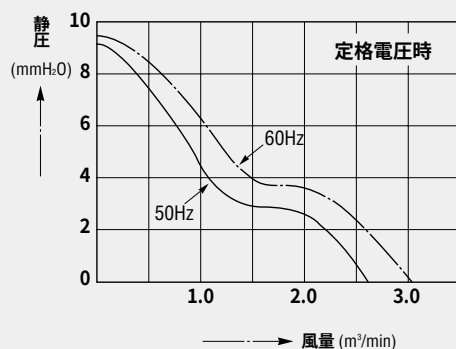
データ（風量－静圧特性）
