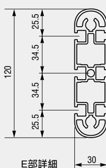
E部詳細
