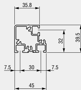
F部詳細
