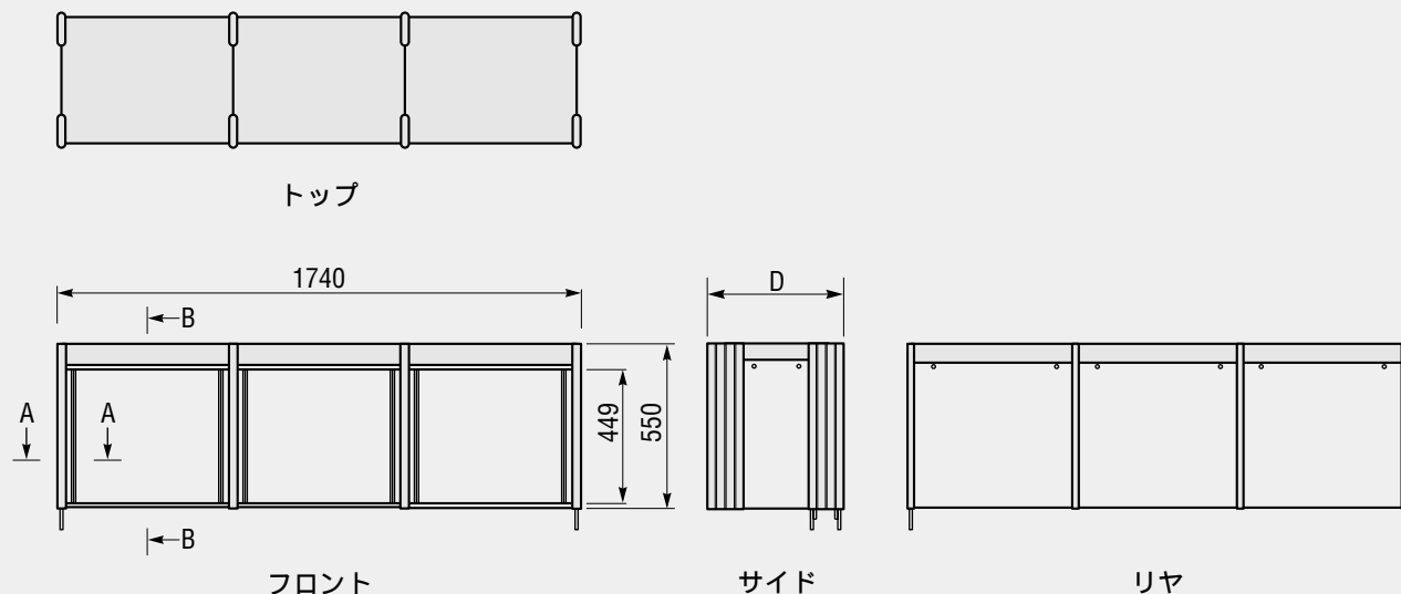
外形寸法図
