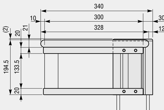
B-B 断面
