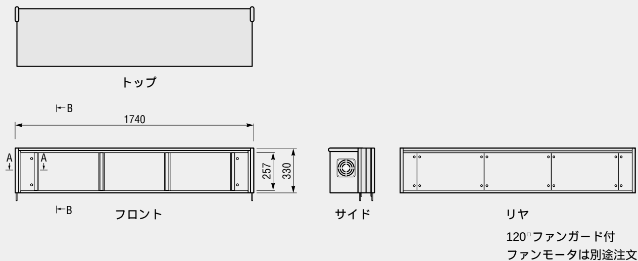
外形寸法図
