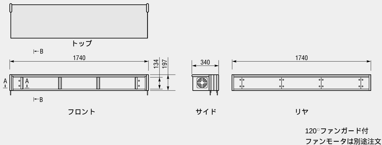
外形寸法図
