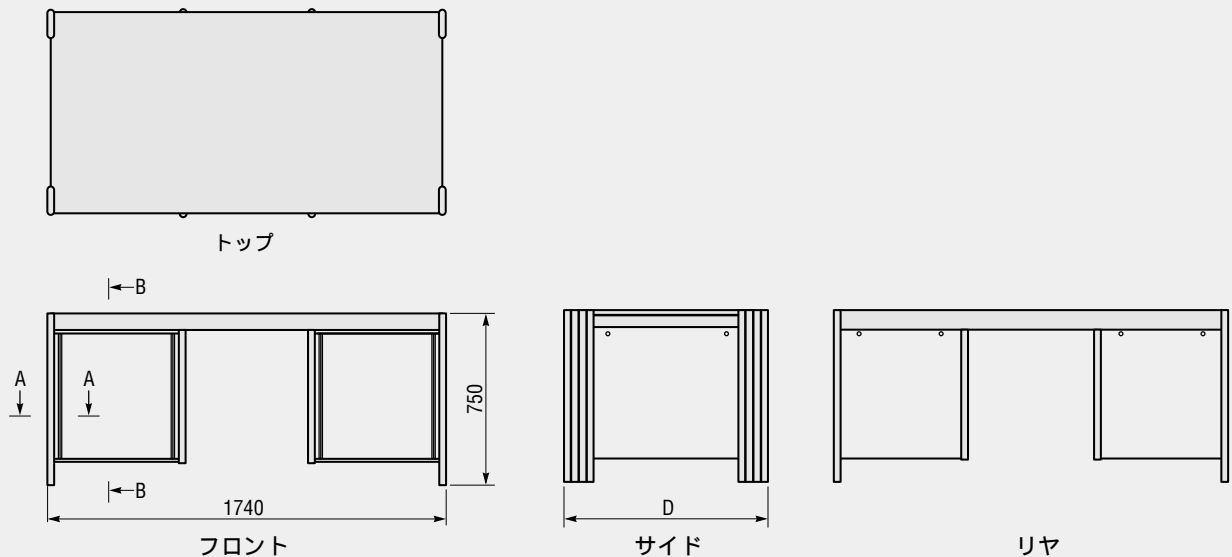
外形寸法図
