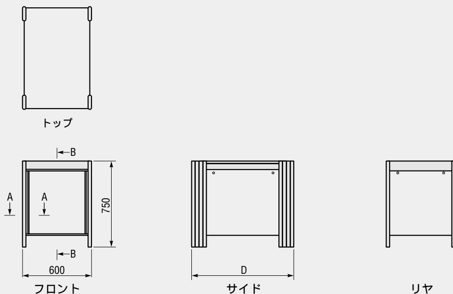
外形寸法図
