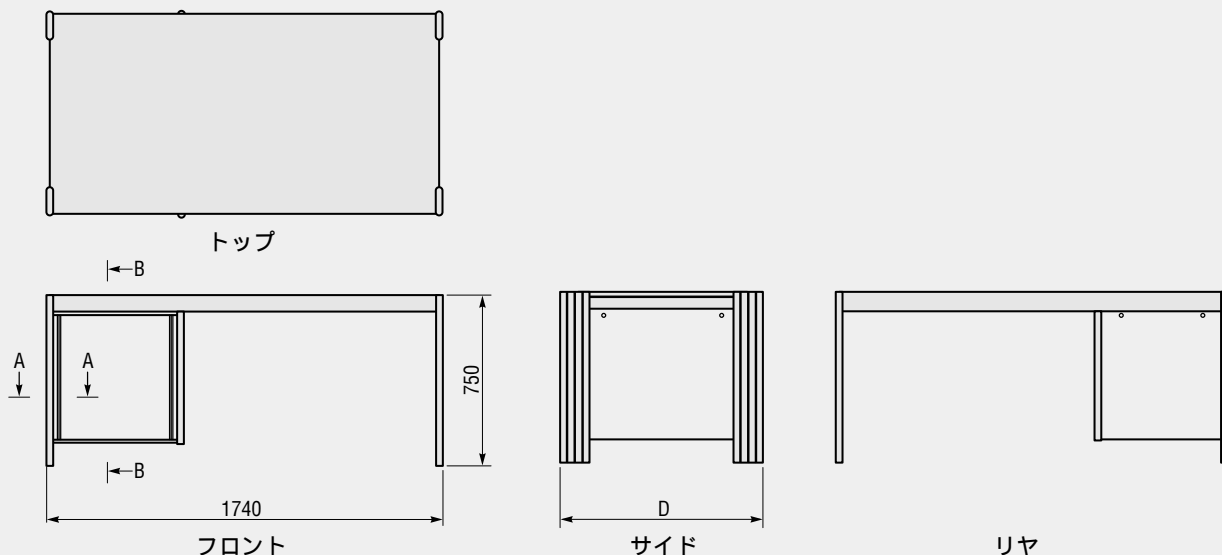
外形寸法図
