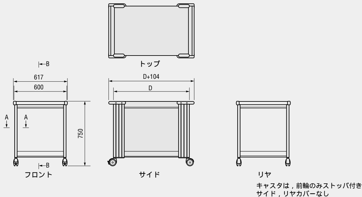
外形寸法図
