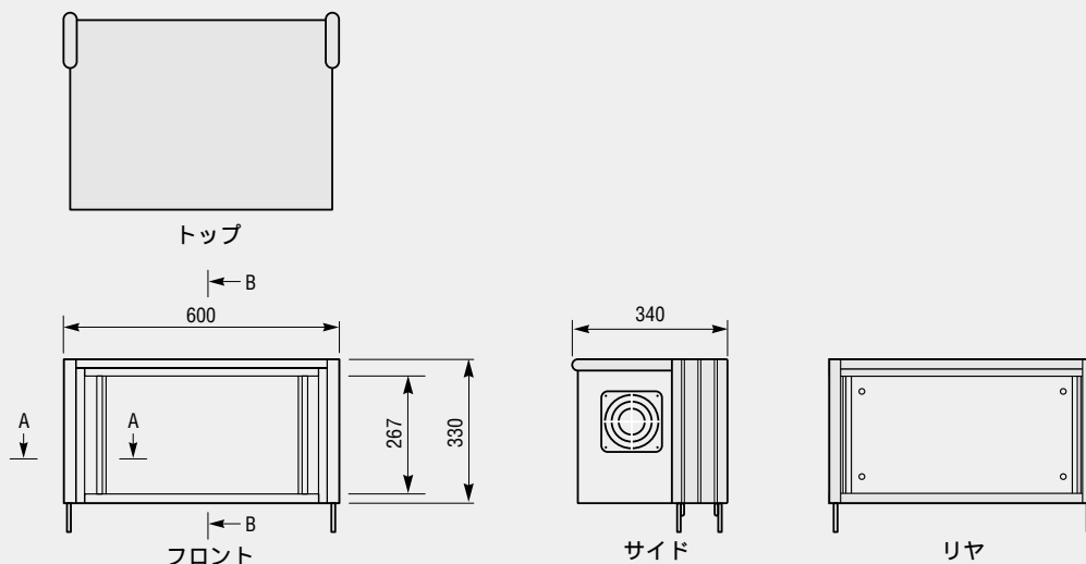
外形寸法図
