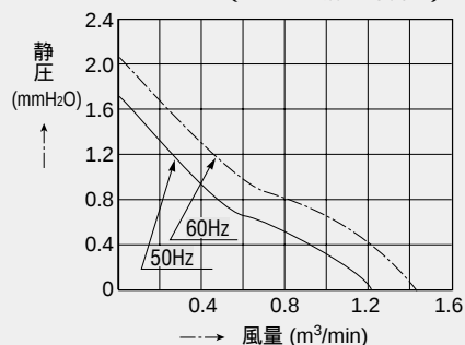
データ（風量—静圧特性）
