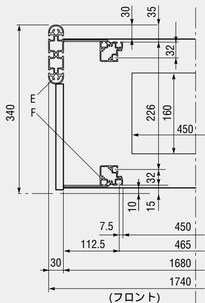
A-A 断面
