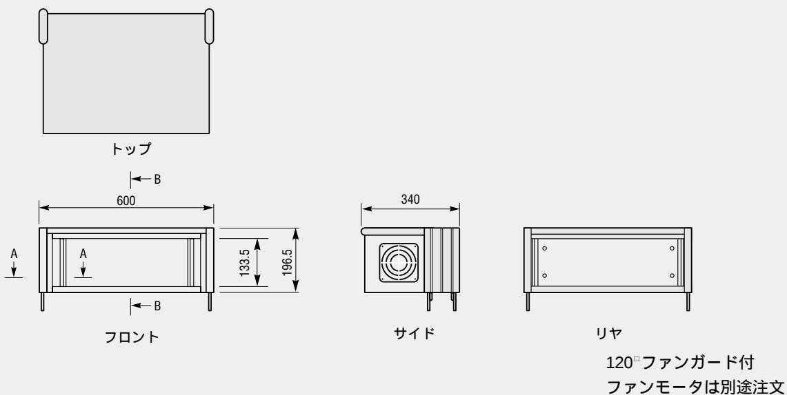
外形寸法図
