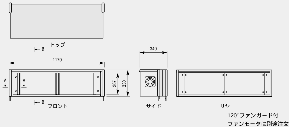
外形寸法図
