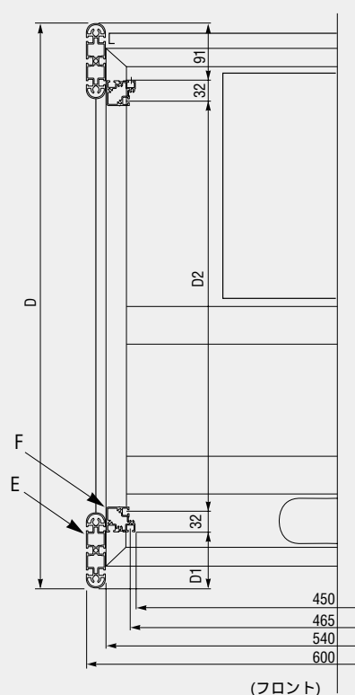
A-A 断面
