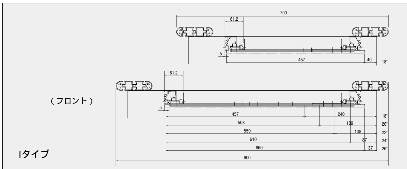
専用スライドレールサポート取付詳細図
