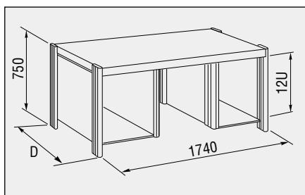
キャビネット両サイド付テーブル W=1740
