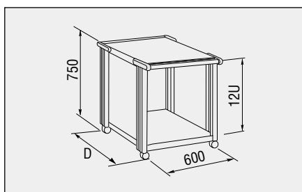
19インチキャビネットワゴン 前後ハンドル付
