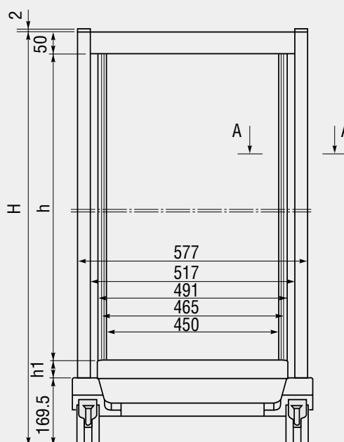
正面図
