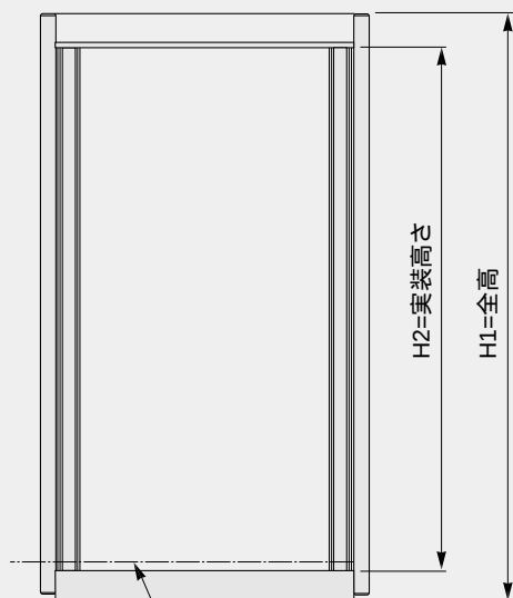
JIS規格変換blankパネル
