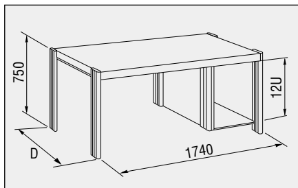
キャビネット右付テーブル W=1740
