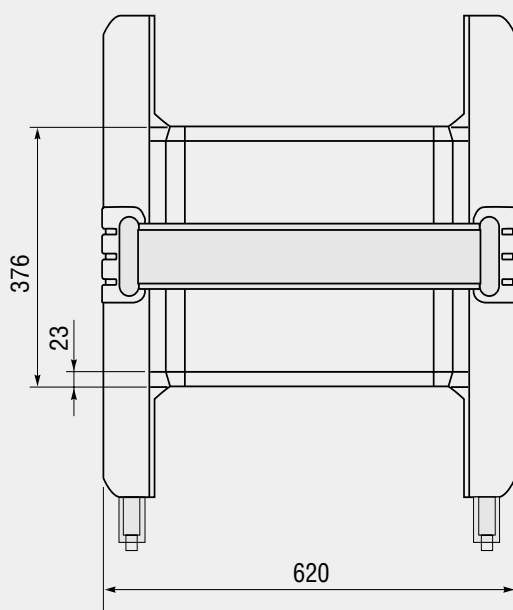
上面図
