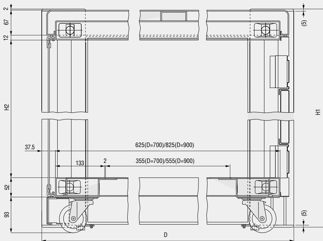
B-B 断面
