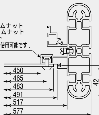
断面A-A
