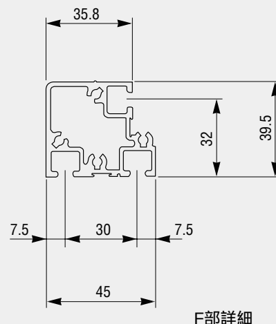
F部詳細
