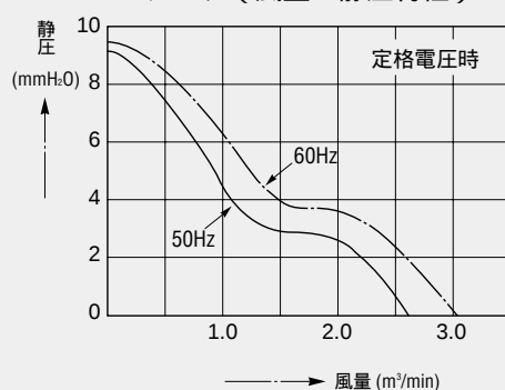
データ（風量 - 静圧特性）
