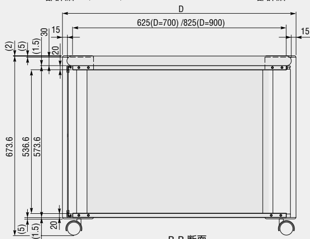
B-B 断面
