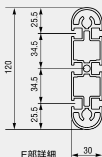
E部詳細
