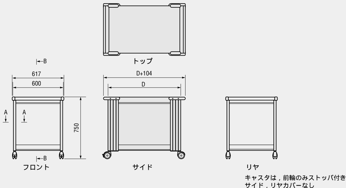
外形寸法図
