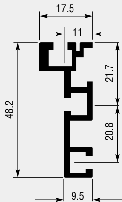
フロント・リヤパネルマウントフレーム
