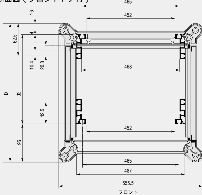
断面図（フロントドア付）
