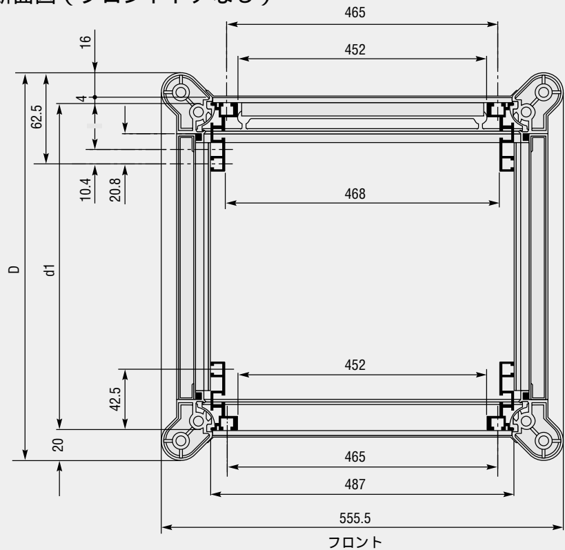
断面図（フロントドアなし）
