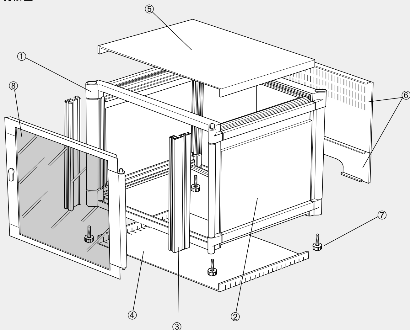
分解図
