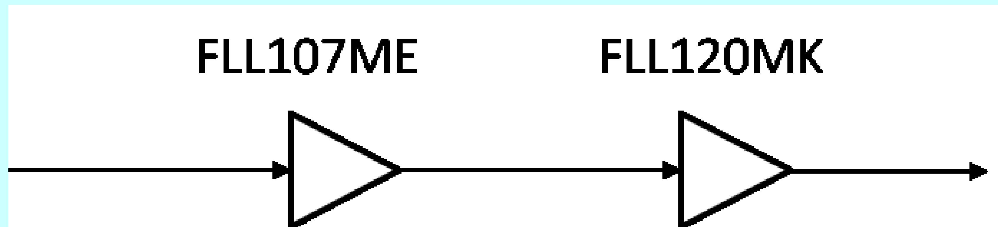
2段直結 高利得・広帯域・平坦 電力増幅器ブロック図
