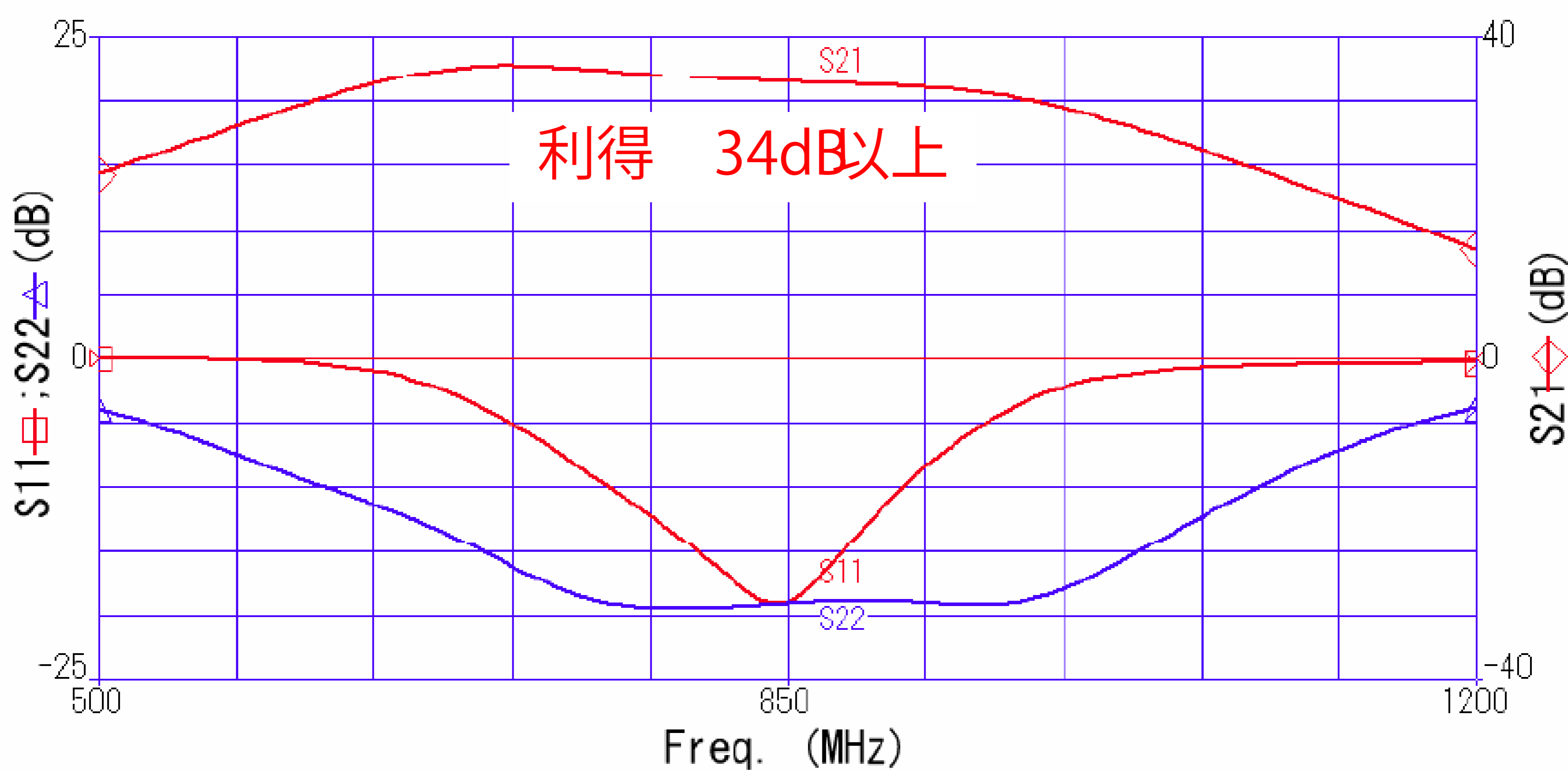
回路シミュレーション周波数特性図
