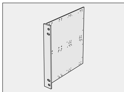
①サイドプレート 材質 A6063S-T5 処理 化学梨地アルマイト
