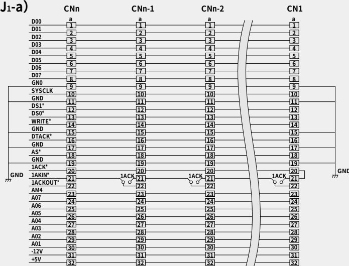
回路図 (J1-a)
