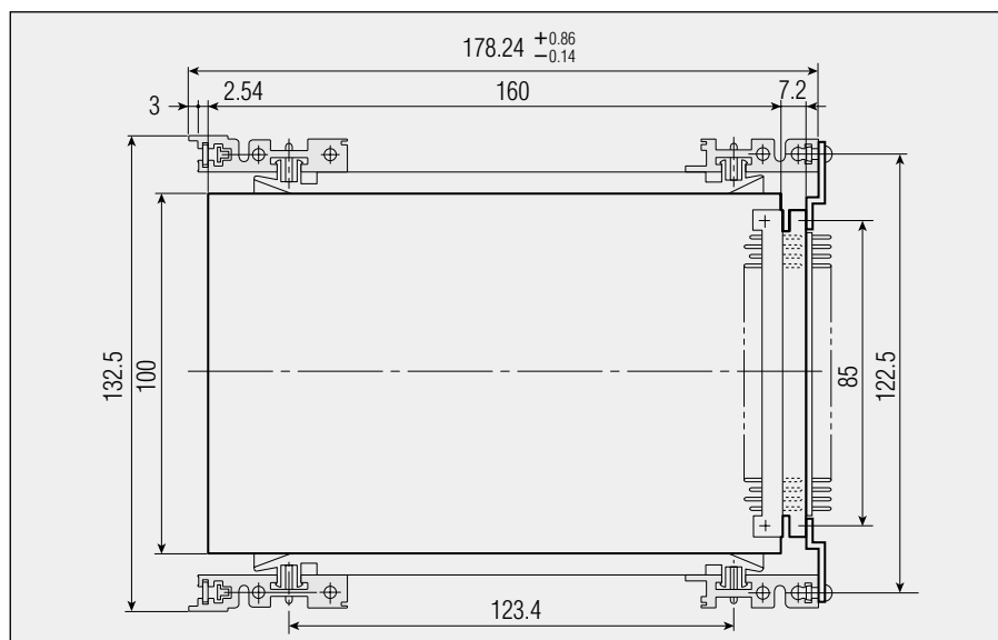
●DIN41617 適合コネクタの 実装構造関係図
