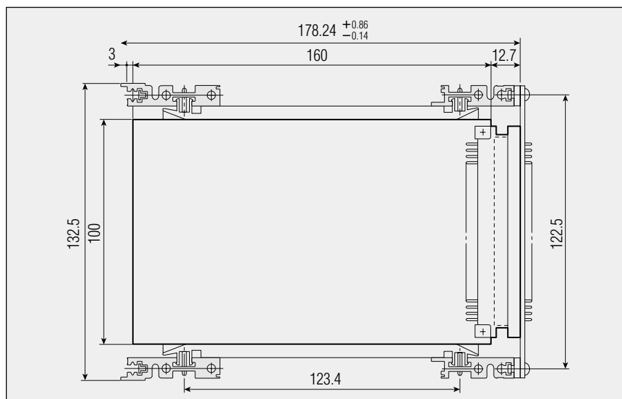
●バックプレーンボードの 実装構造関係図
