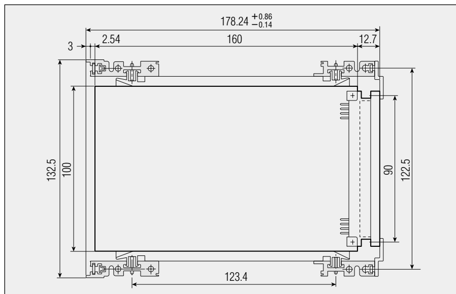
●DIN41612 適合コネクタの 実装構造関係図
