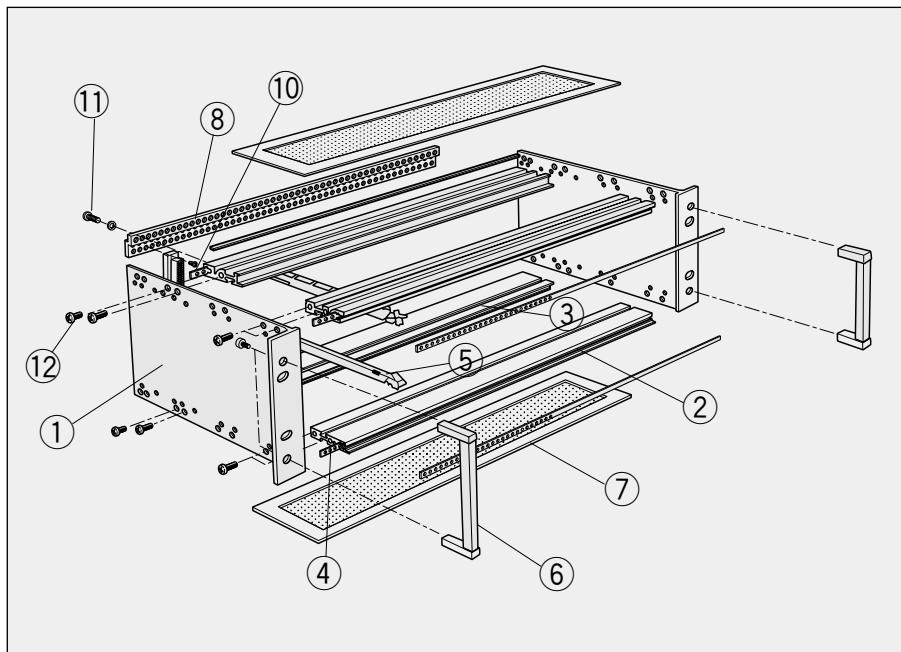
DIN41617を使用する場合の取付図 (参考図)
