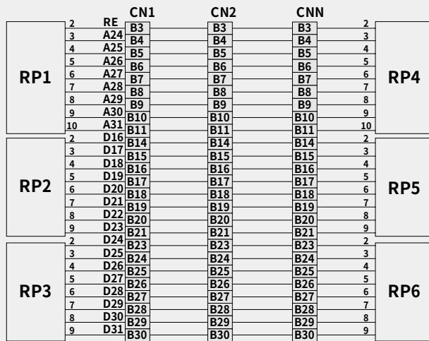
回路図 (J1-I/O-a)
