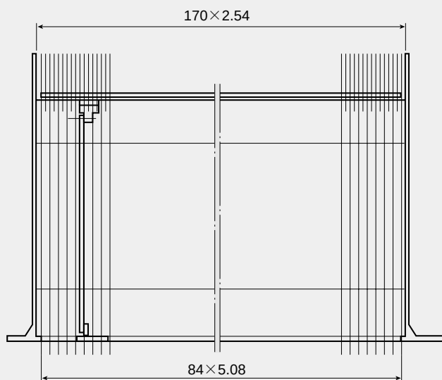
上面図
