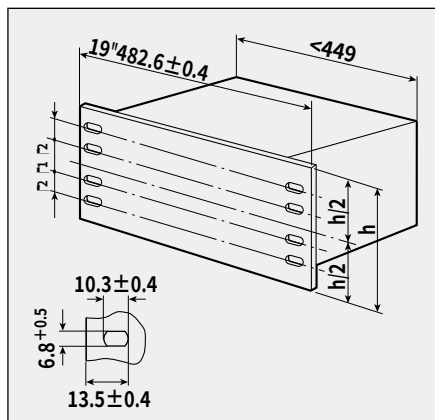
フロントパネル取付寸法図
