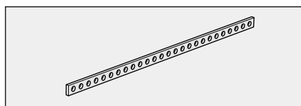
④インサータ 材質 SPCC 処理 MFZn II-C
