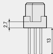
ワイヤーラップターミナル ポスト高さ13mm
