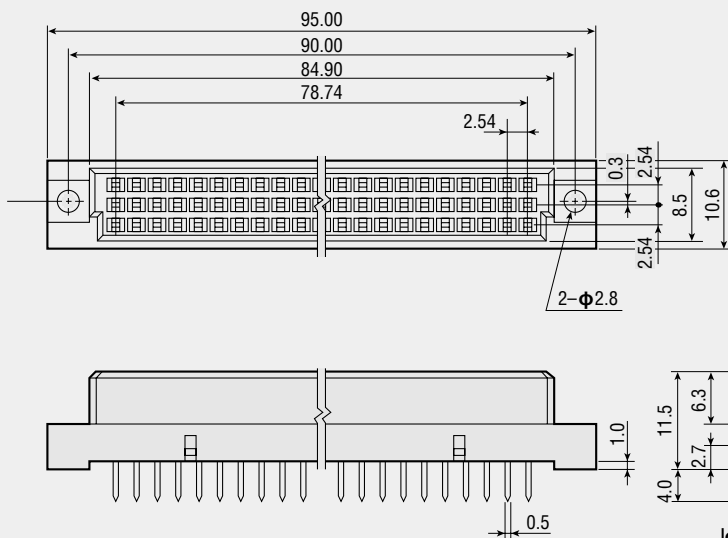
ストレートターミナル ポスト高さ4mm
