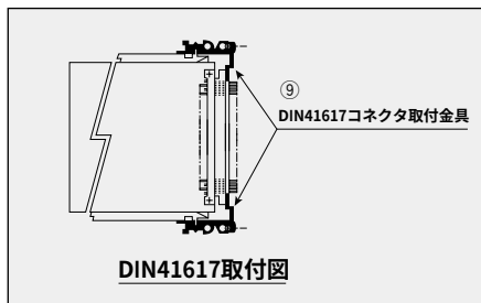
DIN41617を使用する場合の取付図 (参考図)
