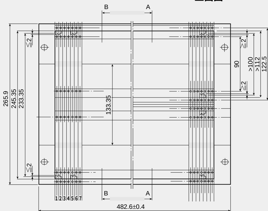
正面図
