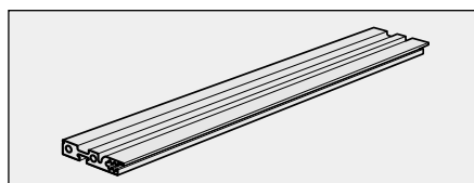
②フロントガイド 材質 A6063S-T5 処理 クロム酸皮膜
