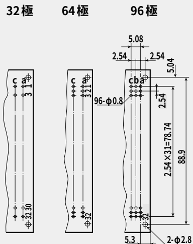
プリント基板穴あけ寸法図 部品面より見た図
