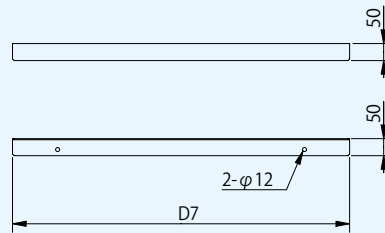
奥行方向受け金具
