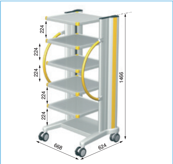
3 compact-cart プロフィ W500 × 40U ■ベーシックフレームプロフィ W500 × 40U 品番: CC.5005.909 ■棚 品番: CC.5020.909 × 5 ■縦型ハンドル 品番: FC.0217.909 × 1
