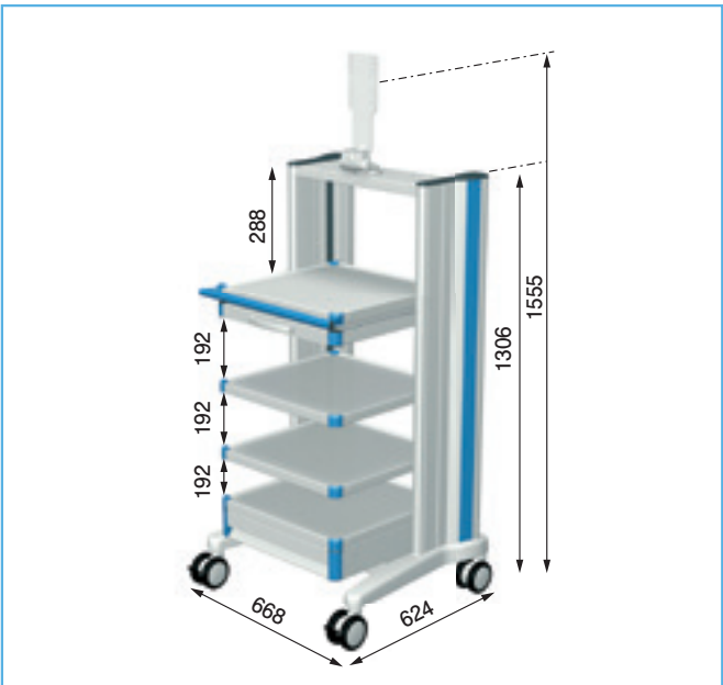
1 compact-cart プロフィ W500 × 35U ■ベーシックフレームプロフィ W500 × 35U 品番: CC.5004.908 ■棚 (ハンドル付) 品番: CC.5021.908 × 1 ■棚 品番: CC.5020.908 × 3 ■キーボード引き出し(マウスパッド付) 品番: CC.5050.908 × 1 ■引き出し3U 品番: CC.5040.908 × 1 ■モニターホルダー 品番: CC.5032.991 × 1
