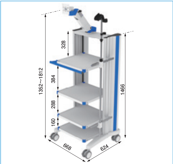
4 compact-cart プロフィ W500 × 40U ■ベーシックフレームプロフィ W500 × 40U 品番: CC.5005.908 ■棚 (ハンドル付) 品番: CC.5021.908 × 1 ■棚 品番: CC.5020.908 × 3 ■標準規格バー 品番: GW.9801.991 × 2 ■内視鏡ホルダー(レールファスナー付) 品番: GW.0868.991 × 1 ■クロスビーム W500 品番: HA.5011.991 × 1 ■Flexion-part (L=300) 品番: HA.2232.908 × 1
