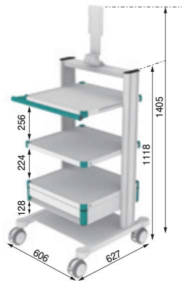
classic-cart エコノミー W500 × 30U
