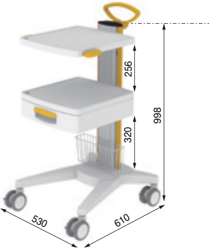
vexio-cart Plus 25U ■ベーシックフレーム (Plus) 25U 品番: JPNT.4051.991 ■ケーブルダクト 25U 品番: NT.4114.909 × 1 ■エレクトロニカルBOX 品番: NT.4121.800 × 1 ■棚 (左右ハンドル付き) 品番: NT.4101.909 × 1 ■引き出し 品番: NT.4104.909 × 1 ■背面ハンドル 品番: NT.2000.909 × 1 ■化粧板 25U 品番: NT.4129.991 × 1 ■バスケット (薄型) 品番: ZV.9892.991 × 1
