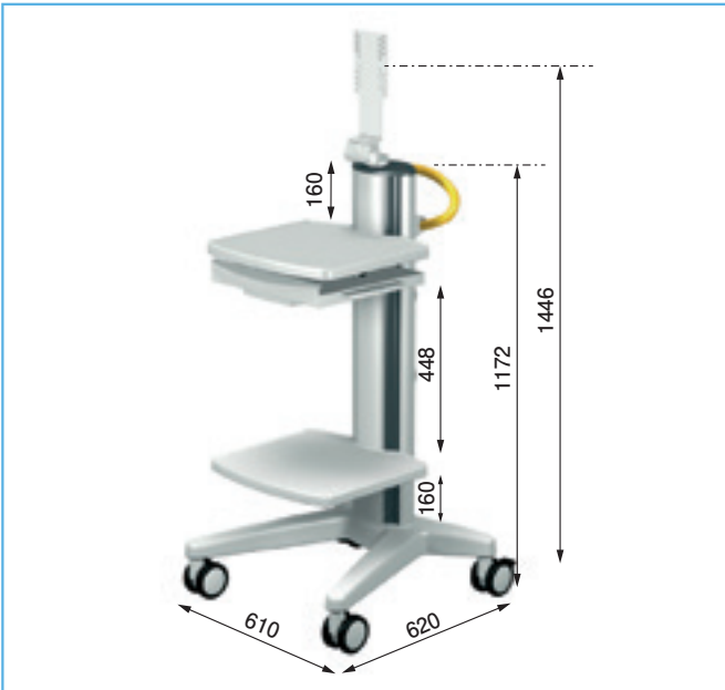
4 pro-cart 30U ■ベーシックフレーム 30U 品番: PT.4001.991 ■プッシュハンドル 品番: PT.2000.909 × 1 ■棚 品番: PT.4100.991 × 1 ■キーボードトレイ 品番: PT.4108.991 × 1 ■モニターホルダ 品番: PT.4118.991 × 1
