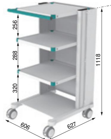
classic-cart エコノミー W500 × 30U
