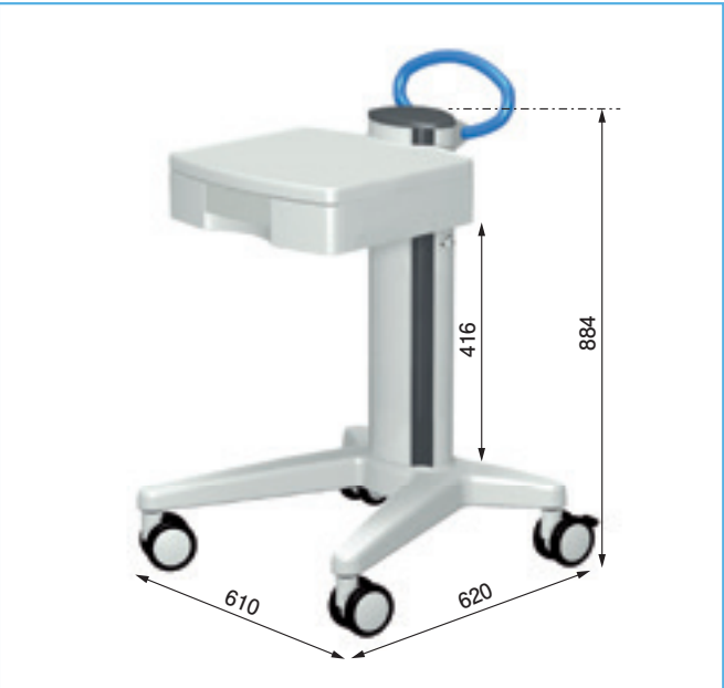
1 pro-cart 21U ■ベーシックフレーム 21U 品番: PT.4000.991 ■プッシュハンドル 品番: PT.2000.908 × 1 ■引き出し 品番: PT.4104.903 × 1
