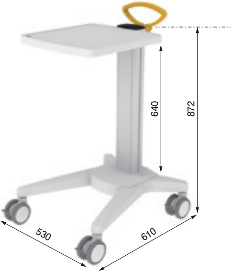
vexio-cart Plus 21U ■ベーシックフレーム (Plus) 21U 品番: NTC.4050.991 ■棚 品番: NT.4100.991 × 1 ■背面ハンドル 品番: NT.2000.909 × 1 ■化粧板 21U 品番: NT.4128.991 × 1
