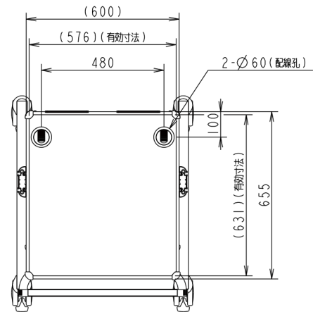
断面 C-C
