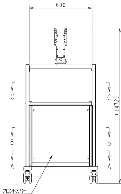
<正面図>
