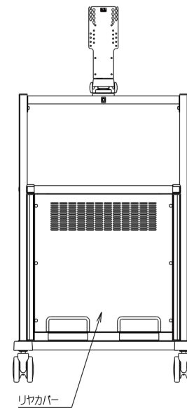
<背面図>
