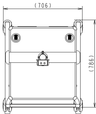
<上面図>
