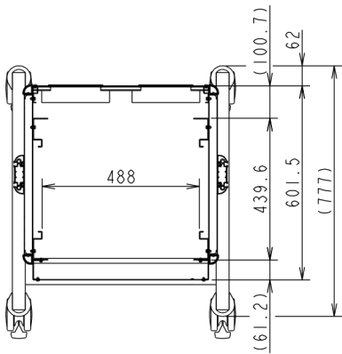
断面 A-A
