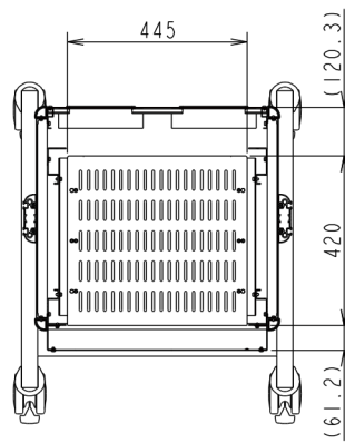
断面 B-B
