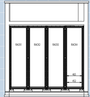
【正面内部断面図】
