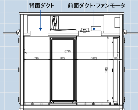
【側面内部断面図】
