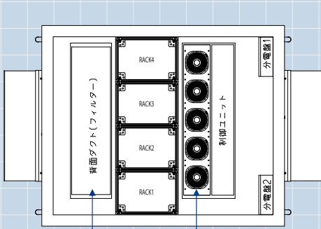
背面ダクト 前面ダクト・ファンモータ
