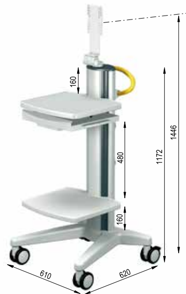
4 pro-cart 30U ■ベーシックフレーム 30U 品番:PT.4001.991 ■プッシュハンドル 品番: PT.2000.909 × 1 ■棚 品番: PT.4100.991 × 2 ■キーボードトレイ 品番: PT.4108.903 × 1 ■モニターホルダ 品番: PT.4118.991 × 1
