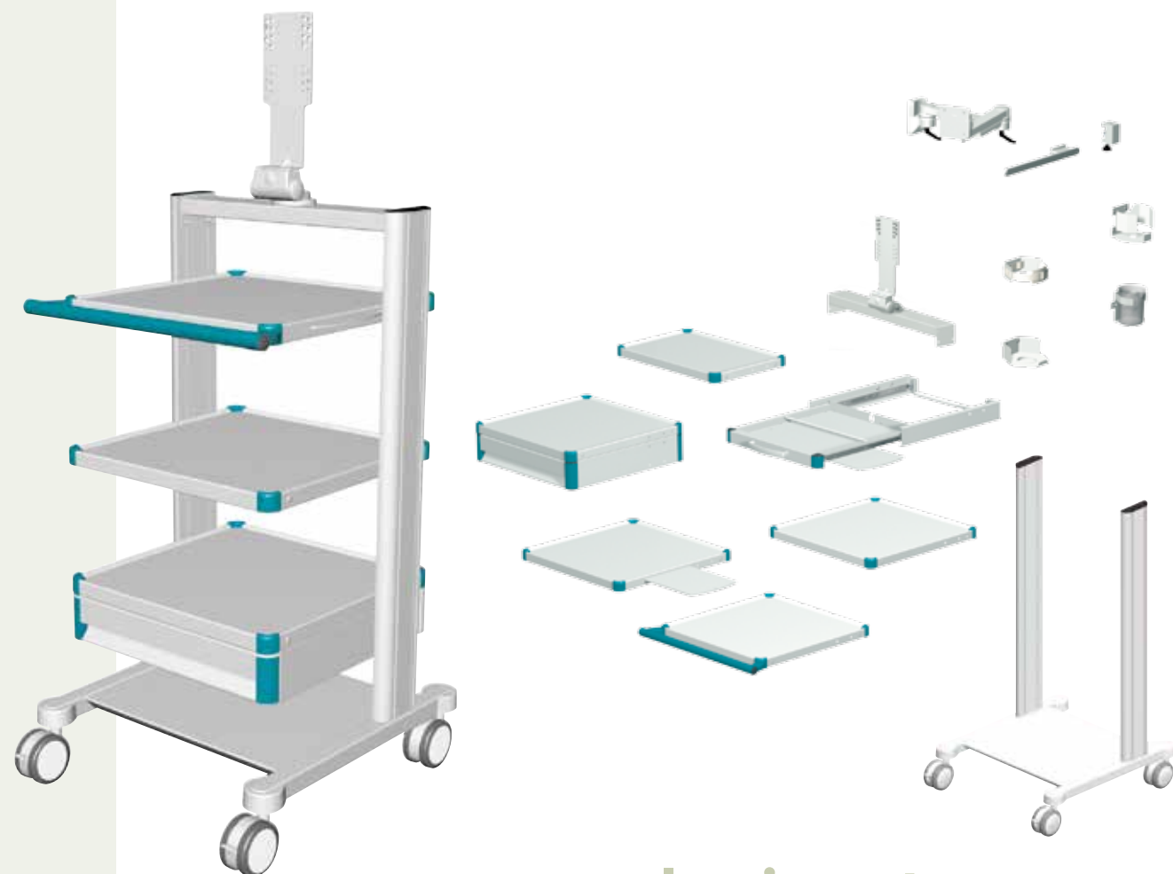
classic-cart モジュールシステム
