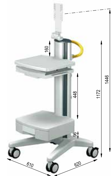
3 pro-cart 30U ■ベーシックフレーム 30U 品番:PT.4001.991 ■プッシュハンドル 品番: PT.2000.909 × 1 ■棚 品番: PT.4100.903 × 1 ■キーボードトレイ 品番: PT.4108.903 × 1 ■引き出し 品番: PT.4104.903 × 1 ■モニターホルダ 品番: PT.4118.991 × 1
