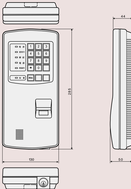
■外形寸法(埋込) (単位:mm)
